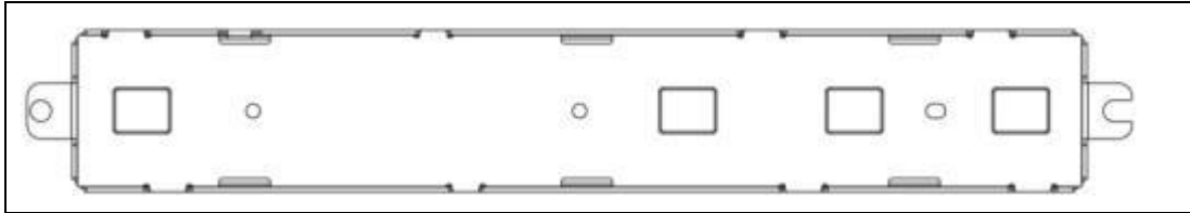
Figure 7-9. Bottom Stiffener Depth Module D450
